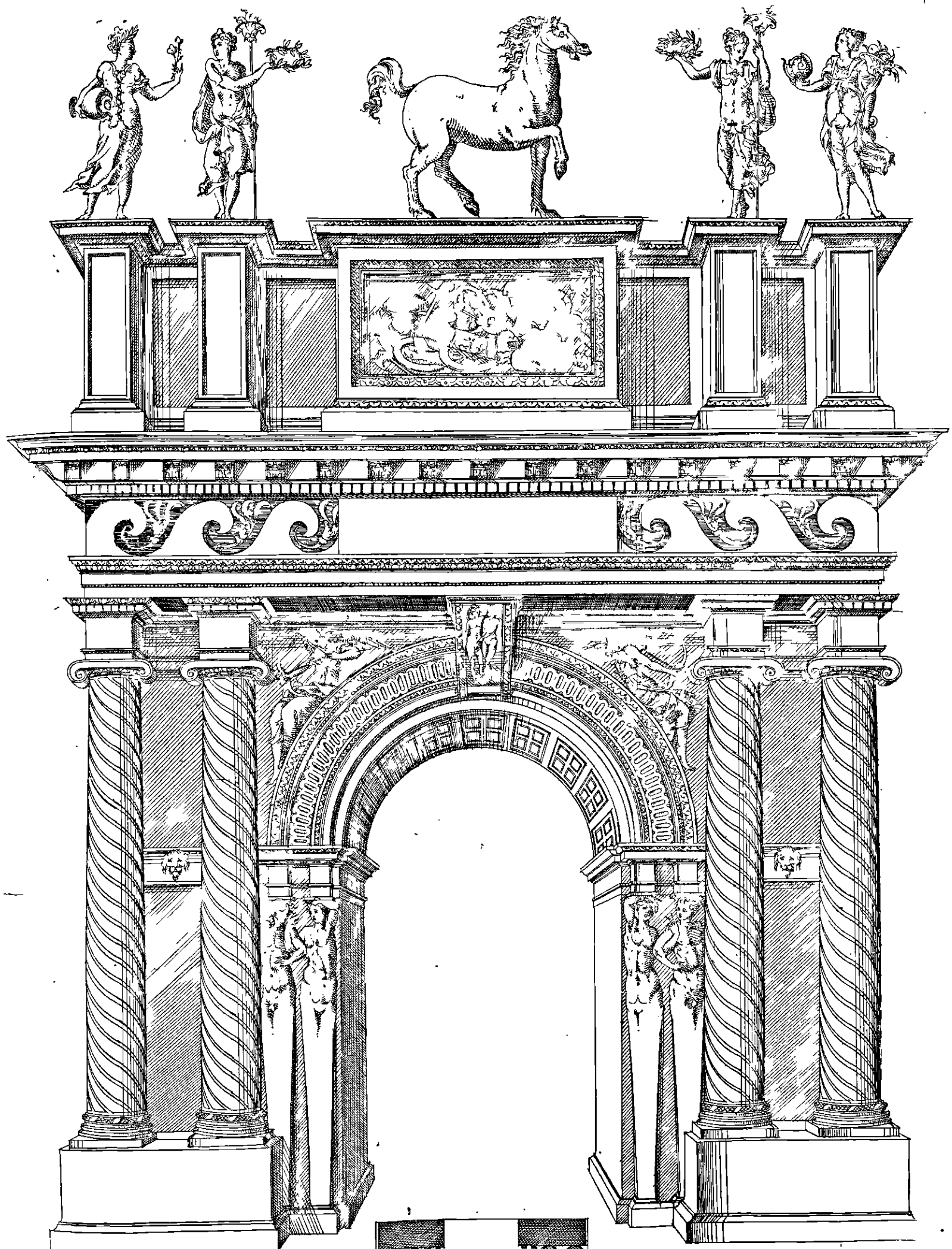
ARC SELON LORDRE IONIQUE
