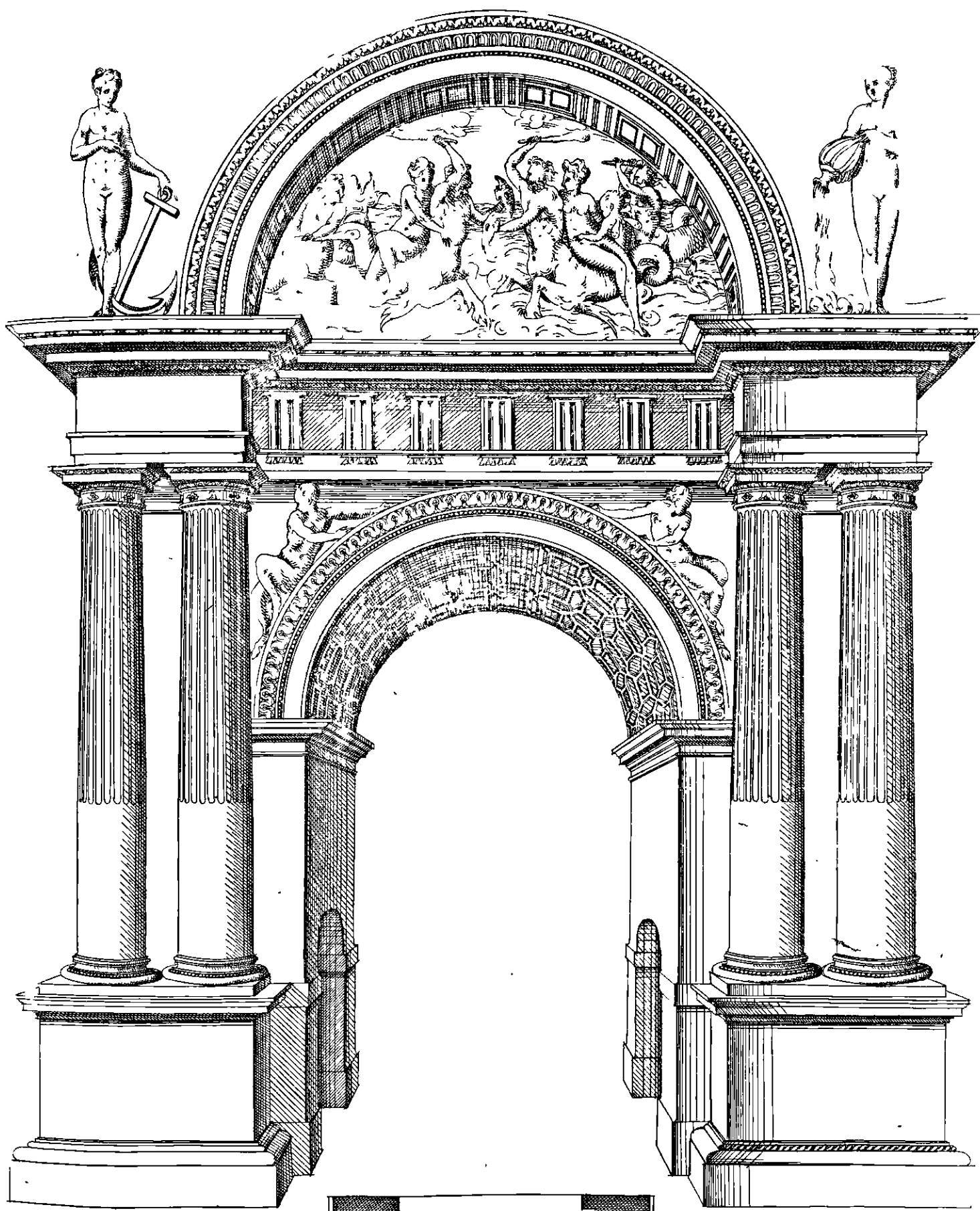
ARC SELON L'ORDRE DORIQUE
