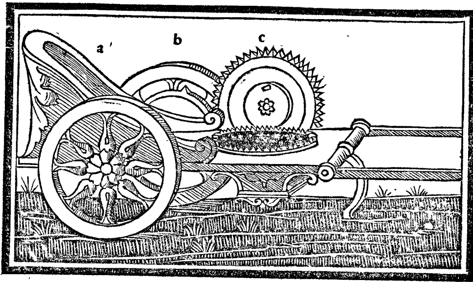
Rheda a: capsū rhe- de b: rota c: tympanū Reliqua itel- liguntur ex lectione
