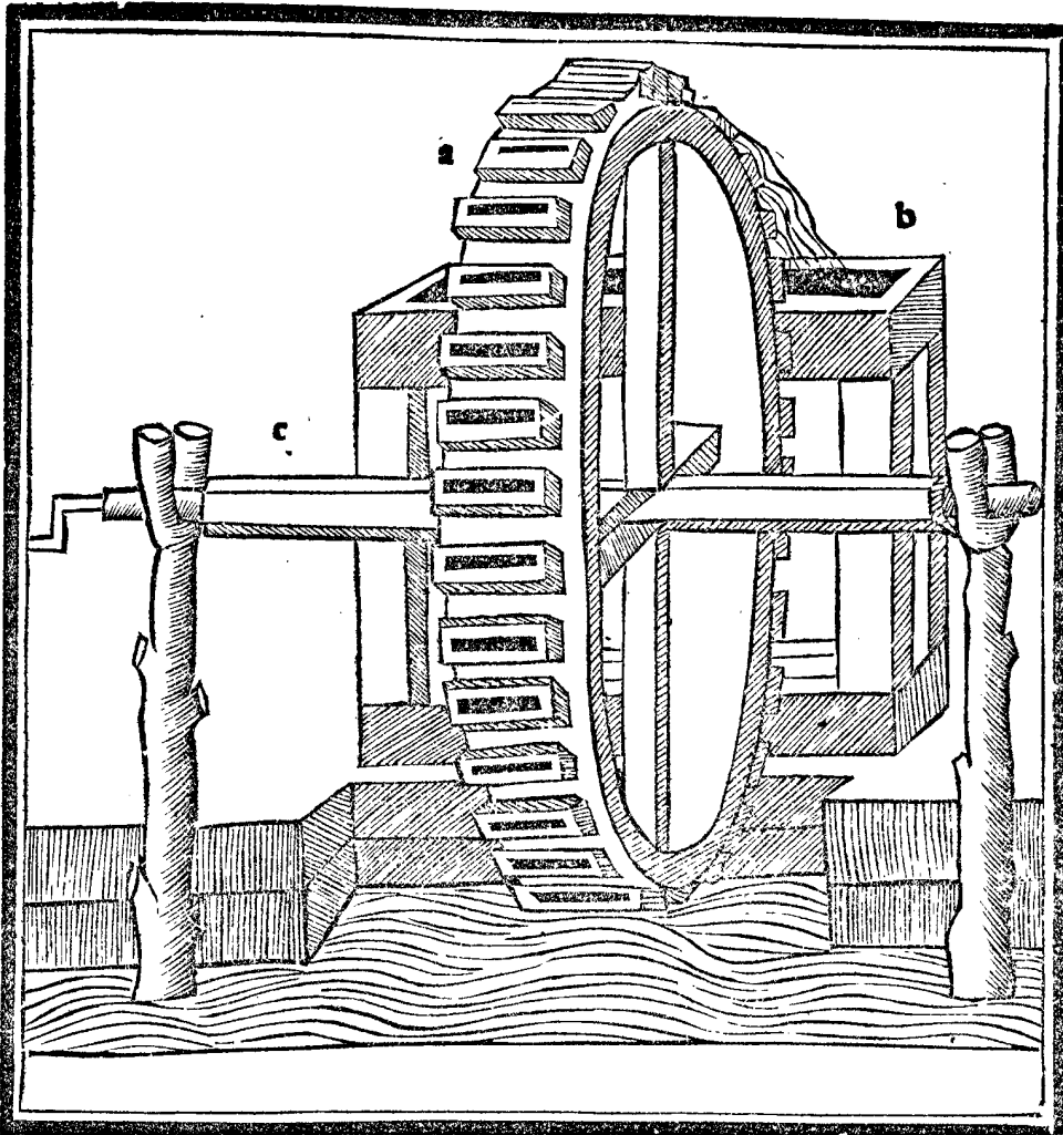
a. modiolii b. castellū c. axis
