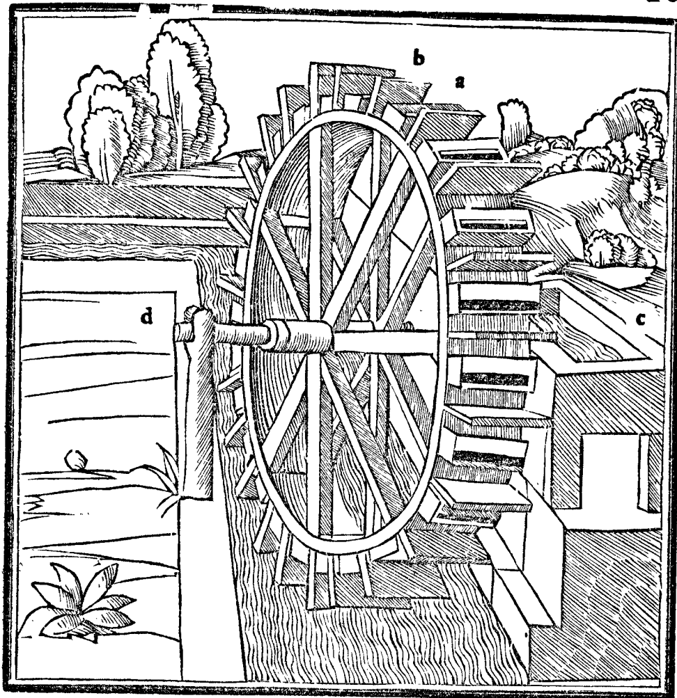
a. modiolus b. pinne : hæ nãq̃ alterna tim positæ sunt cū mo- diolis. c. castellum d. axis
